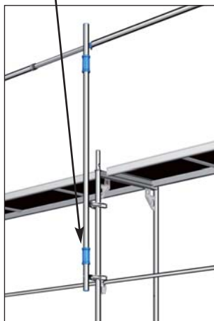
Rys. 12 i 13: Podłączenie słupka montażowego do ramy pionowej Blitz
