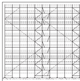
Rys. 36: Ułożenie stężeń
