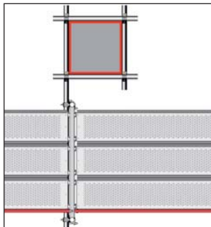
Rys. 47: Zakotwienie do podpory betonowej
