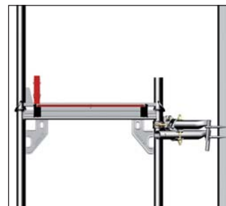
Rys. 45: Kotwa V, widok z boku
