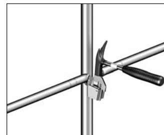
Rys. 21: Utwierdzenie poręczy
