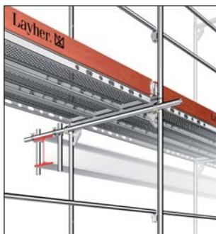
Rys. 48: Zakotwienie do belki poziomej
