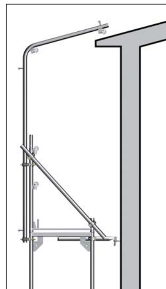
Rys. 103: Sposób montażu podpory planeki ochronnej
