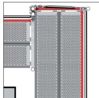
Rys. 57: Widok z góry
