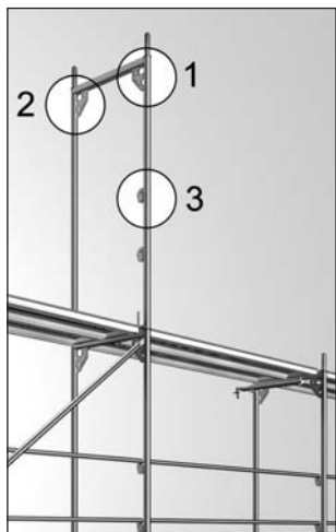
Rys. 7: Punkty zaczepienia 1 i 2
